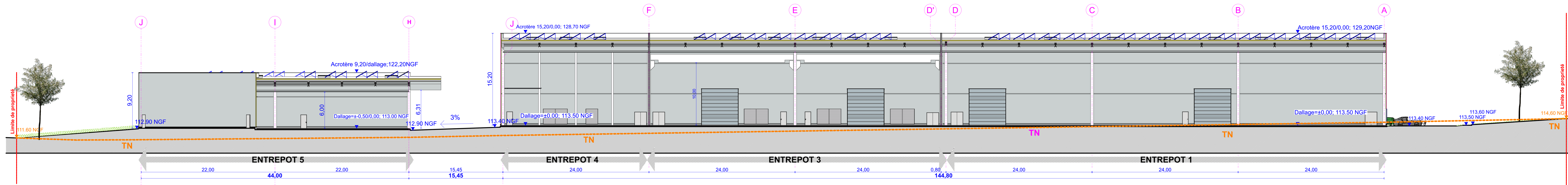
COUPE BB
