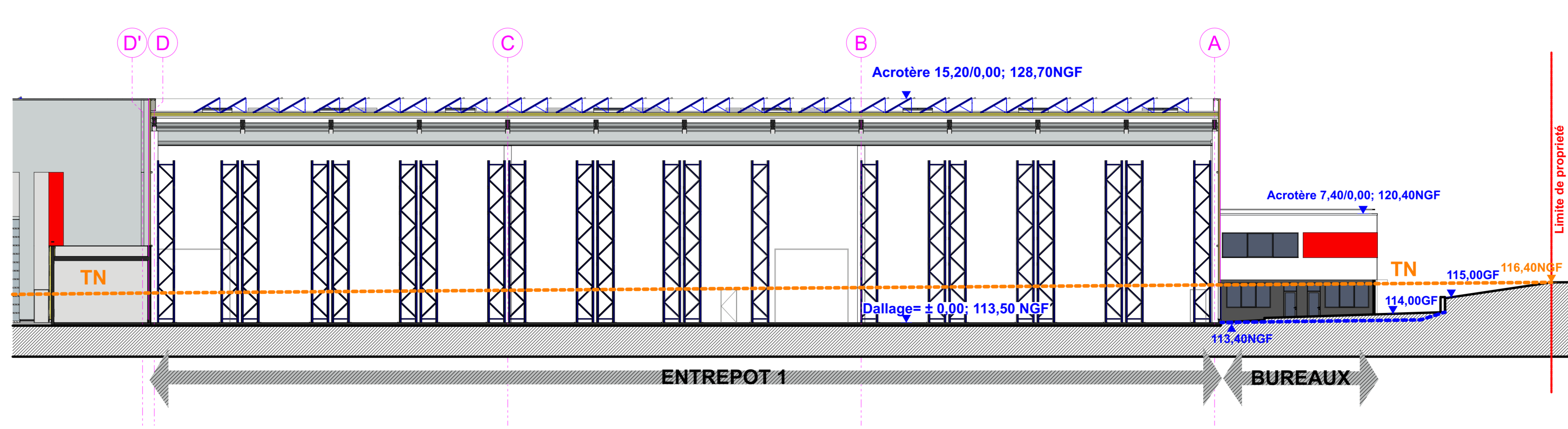
COUPE DD
