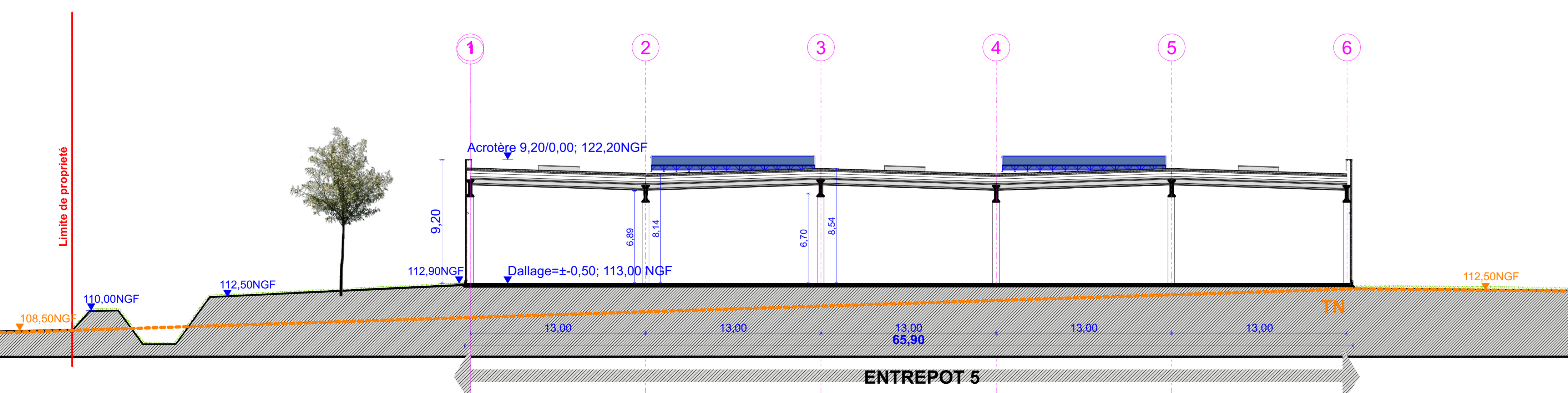
COUPE CC
